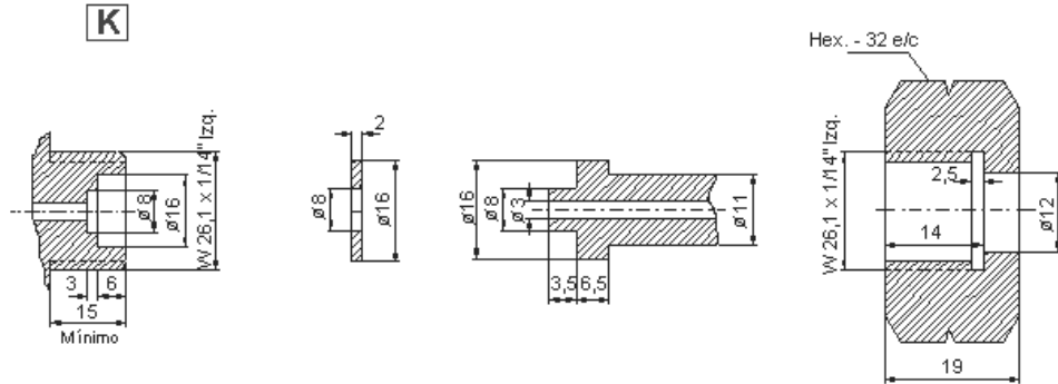
ACOPLAMIENTO W 26,1 - 14 Hilos/Pulgada (IZQUIERDAS) TIPO ALTAMENTE CORROSIVOS
