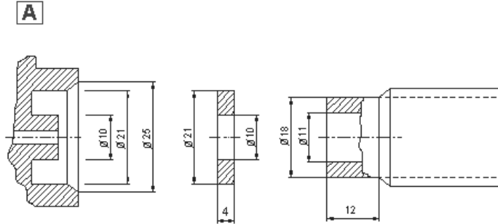
ACOPLAMIENTO DE ESTRIBO TIPO ACETILENO Gases: Acetileno: C 2 H 2
