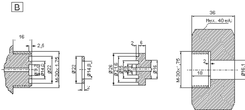
ACOPLAMIENTO M 30 x 1,75 METRICO (DERECHAS) TIPO AIRE Gases: Aire natural Aires sintéticos
